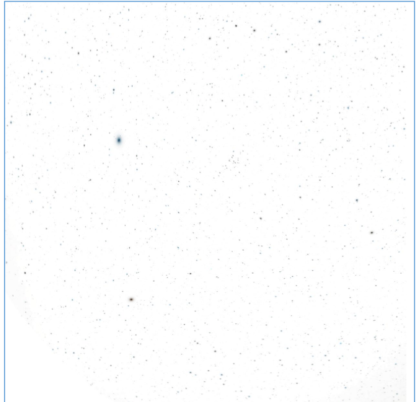
Ein Ausschnitt des Frühlingssternhimmels
